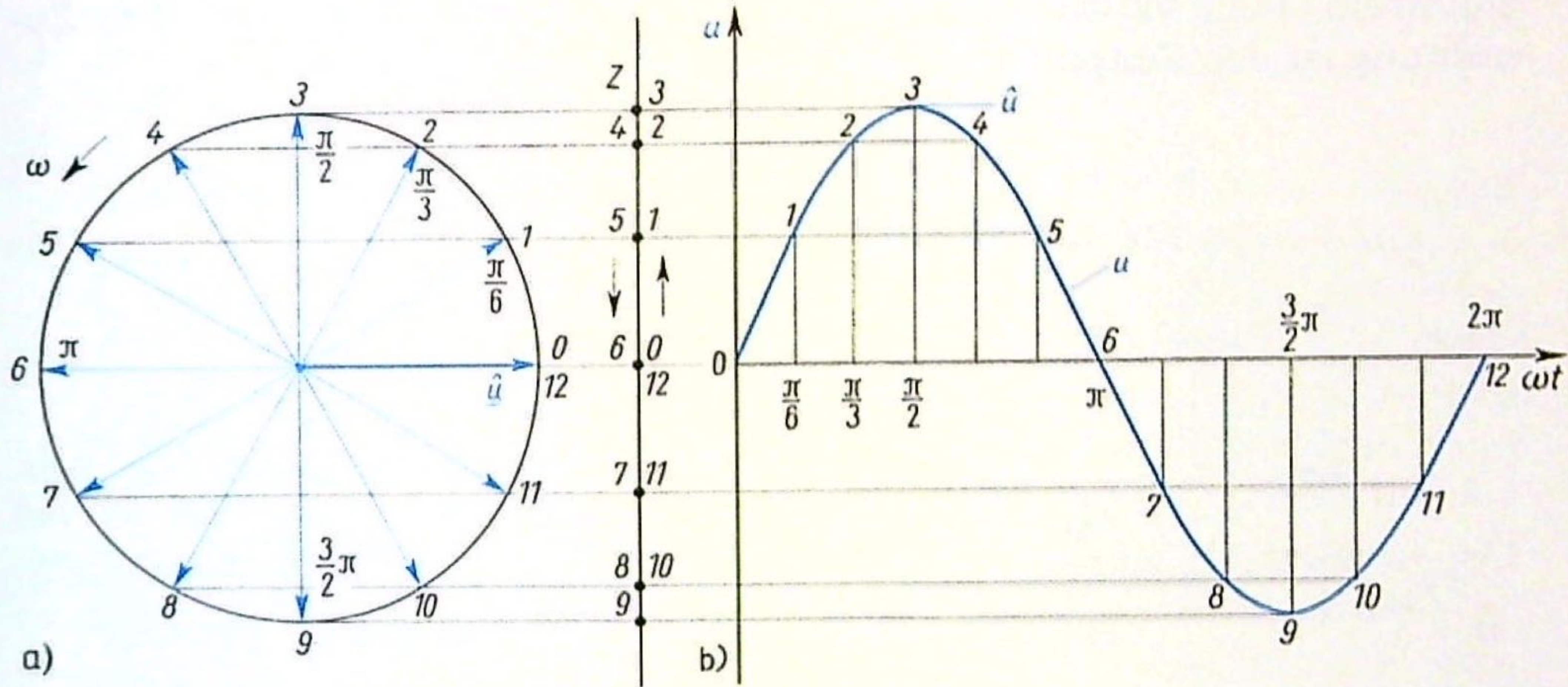
3.6 Zusammenhang zwischen Zeigerdiagramm (a) und Zeitdiagramm (b) Z Zeitlinie
